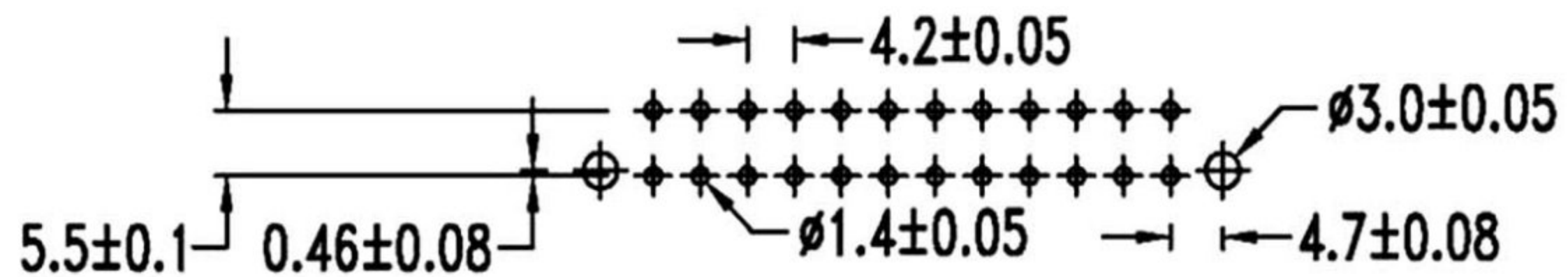
P.C.B. hole dimensions
