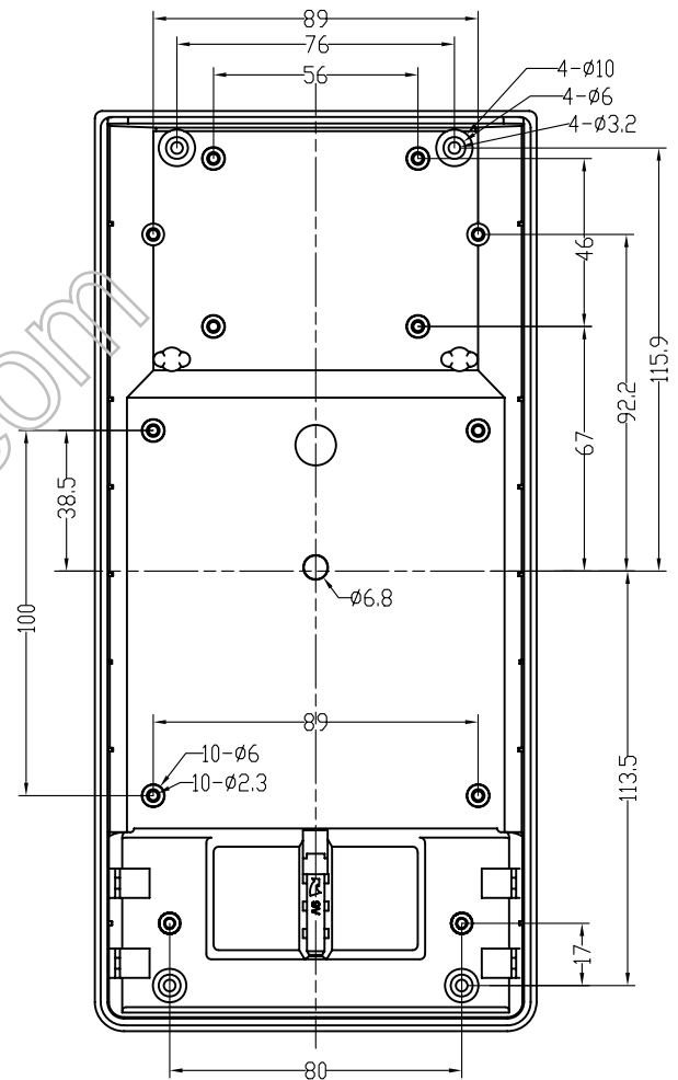
下盖正视图
